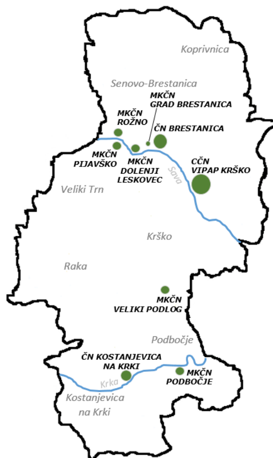
Slika 8: Prikaz ČN in MKČN, ki so v upravljanju Kostak, d. d.
